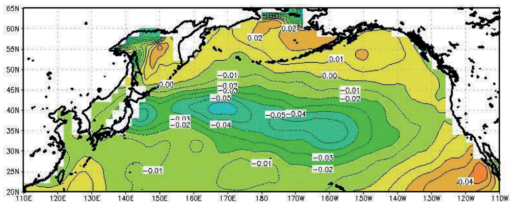
Рис. 10. Величины линейных трендов ( ^{\circ}\text{C}/\text{год} ) средних значений зимних аномалий ТПО в Северной Пацифике в период 1946–1981 гг. (холодный период).
