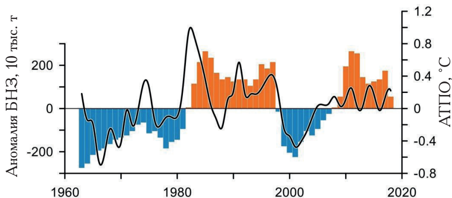
Рис. 7. Динамика аномалий биомассы нерестового запаса минтая северной части Охотского моря (БНЗ, столбики) и средних зимних аномалий температур поверхности Охотского моря (АТПО, линия).
