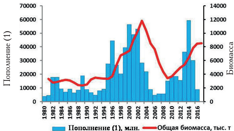
Рис. 32. Динамика общей биомассы путассу и численность пополнения в возрасте 1 год (ICES, 2017). Годы на оси абсцисс соответствуют годам нереста.
