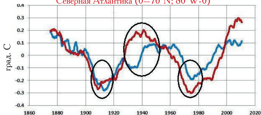
Рис.4. Аномалии температуры поверхности океана в северных частях Атлантического и Тихого океанов (АТПО) в 1870–2015 гг. после удаления линейного тренда (Tisdale, 2015).
