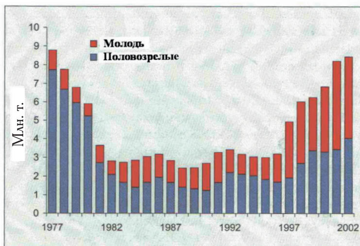
Рис. 33. Динамика общего запаса пугассу в Северной Атлантике, 1977–2002 гг. (The Norwegian Sea ..., 2004).
